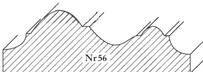
Nr 56 27x80 Furu B.
