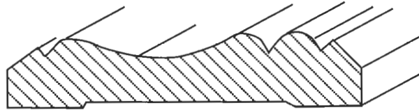
D21 14x67 Dekorlist
