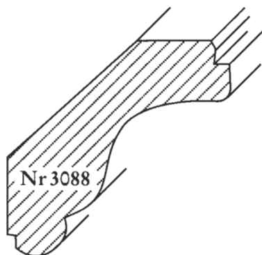
Nr 3088 Allmoge Taklist 19x53 Furu A.
