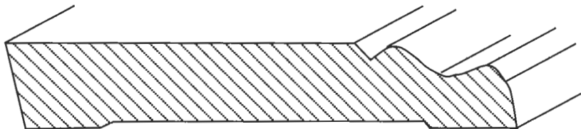
S6 15x95 Sockellist
