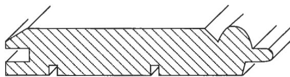
Pärlspont 14x70 Furu B
