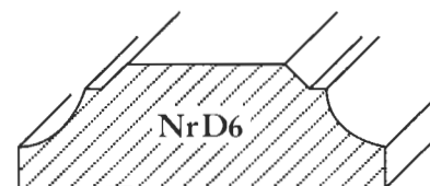
Nr D6 15x44 Furu A.
