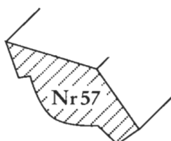
Nr 57 Takbrottslist för snedtak 10x30 Furu A.
