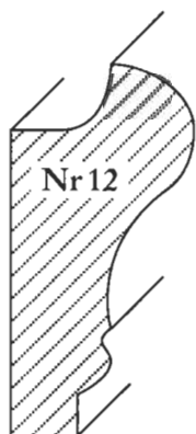
Nr 12 Tavelhängarlist 22x45 Furu A, Vitmålad. (Krokarfinns)
