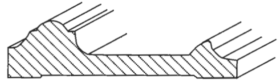
D22 15x60 Dekorlist
